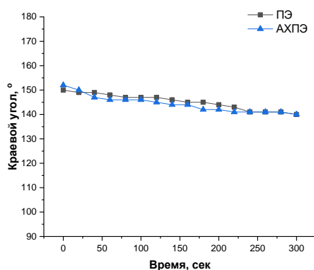
Рис. 1б. График зависимости краевых углов смачивания от времени для тканей с нанесенным на них \text{CF}_3 -полимером после отжига (б).
